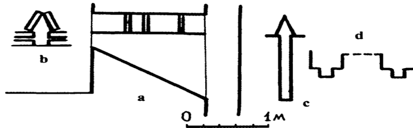
16-рasm. Қизилқалъа тарҳи деталлари: а) шинак кесмаси; б) туйнукнинг кириши; с) туйнукнинг чиқиши; д) шимоли-ғарбий девордаги пиястрлар
