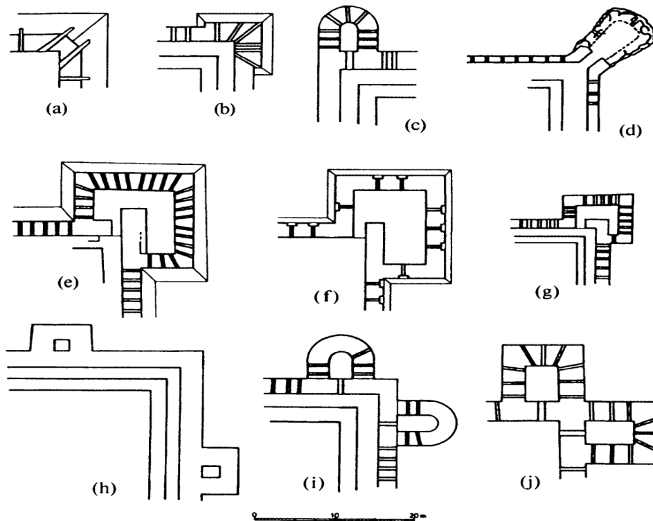
81-рasm. Бурчаклар ҳимояси: а) Жонбосқалъа; б, с, и) Қўрғошинқалъа; д) Бозорқалъа; е) Оқшaxonқалъа; ф) Тупроққалъа; г) Анқақалъа; ҳ) Хивадаги Тупроққалъа; ж) Катта Қирққизқалъа
